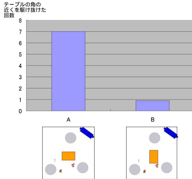
図 9: 駆け抜けタイプのシミュレーション結果
