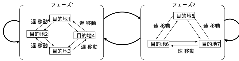
図 2: 移動モデルの例
