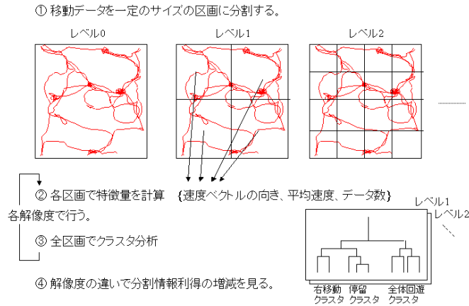
図 7: 多解像度クラスタ分析法
